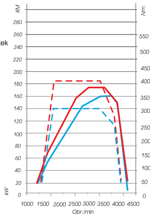
F1CE5+ 170 hp
